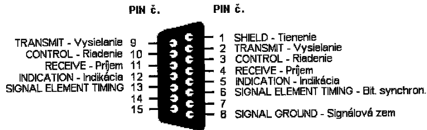
Obr. č. 1: Konektor rozhrania X.21
