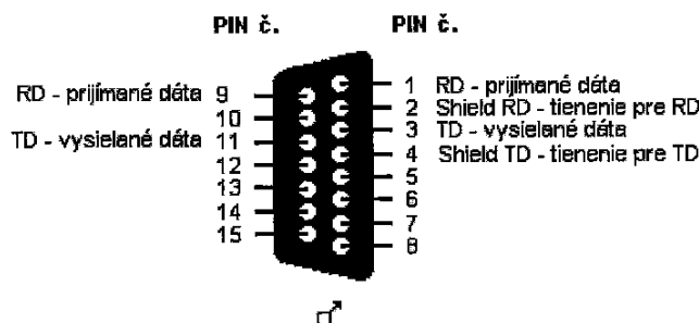
Obr. č. 3: 15 pinový konektor rozhrania G.703 – DB-15F
